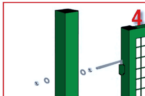
4 - Regolare le cerniere agendo sulle viti
